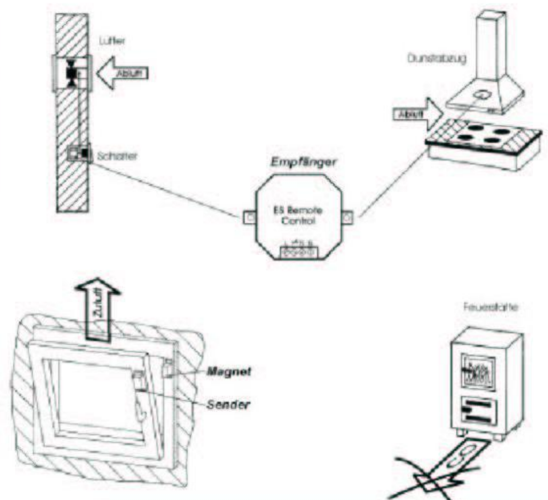
Bild 3 Fensterkontaktschalter drahtlos (FUNK)
