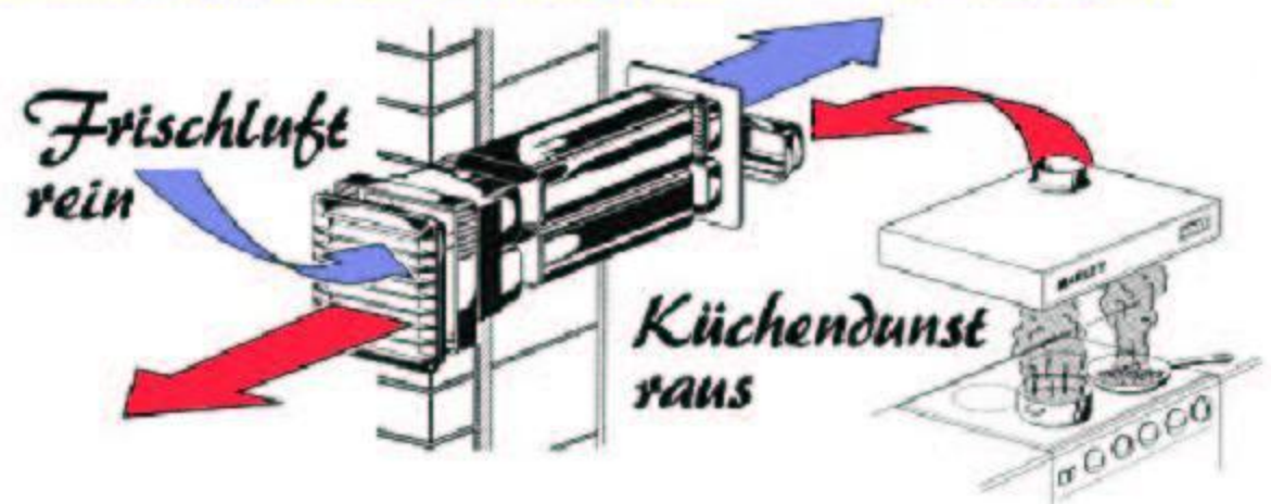
Bild 1 kombinierter Abluft/Frischluft Mauerkasten
